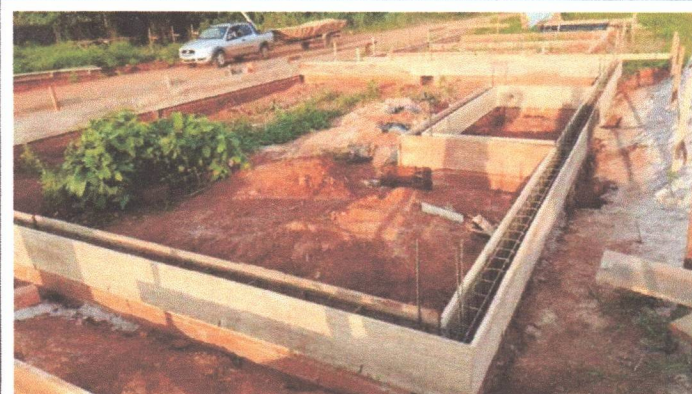
VIGAS BALDRAME
