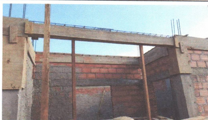
ALVENARIA, ARMAÇÃO VERGAS CONTRA VERGAS
